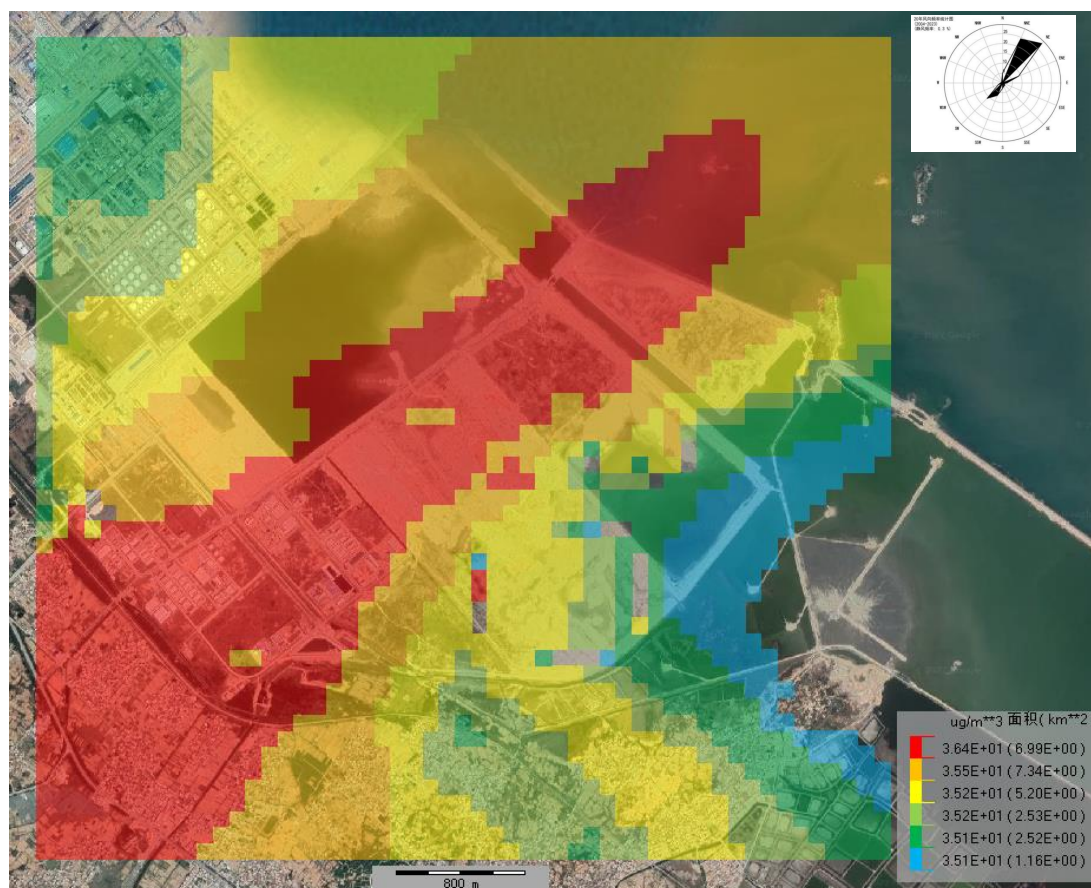
图 6.2-17 NO 2 叠加在建拟建和现状背景保证率下日平均浓度网格分布图
