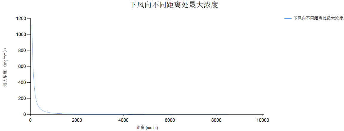
图 7.5-4 硫化氢泄漏事故下风向不同距离处硫化氢的最大浓度图（最常见气象条件）
