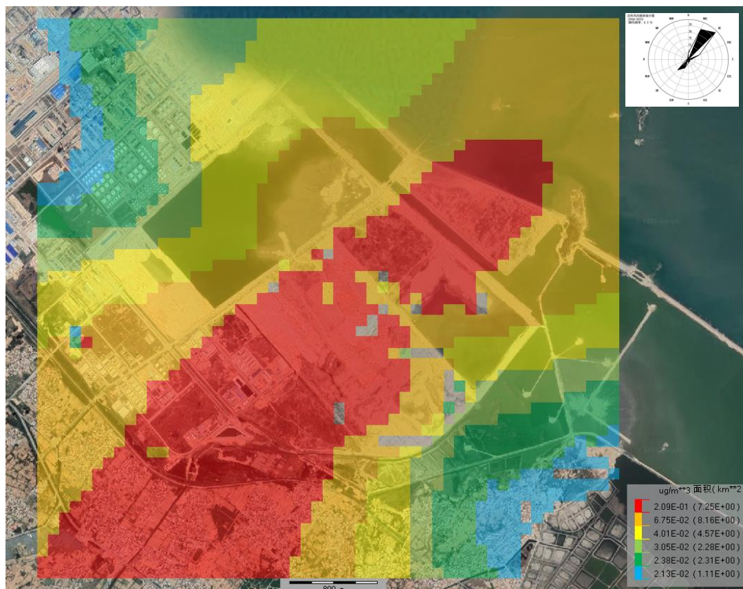
图 6.2-8 \text{SO}_2 年均浓度网格分布图
