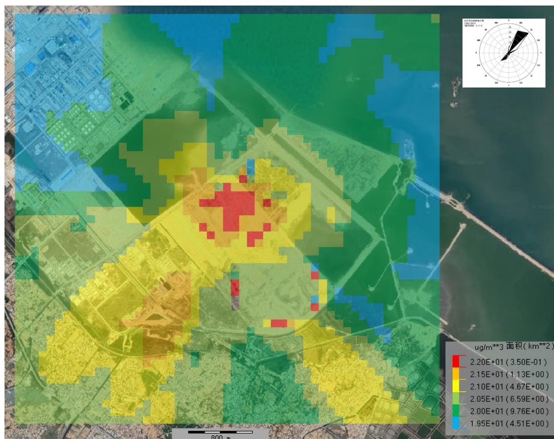
图 6.2-21 硫酸叠加在建拟建和现状背景值后小时平均浓度网格分布图
