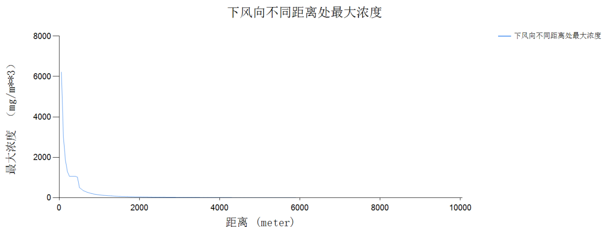
图 7.5-1 硫化氢泄漏事故下风向不同距离处硫化氢的最大浓度图（最不利气象条件）
