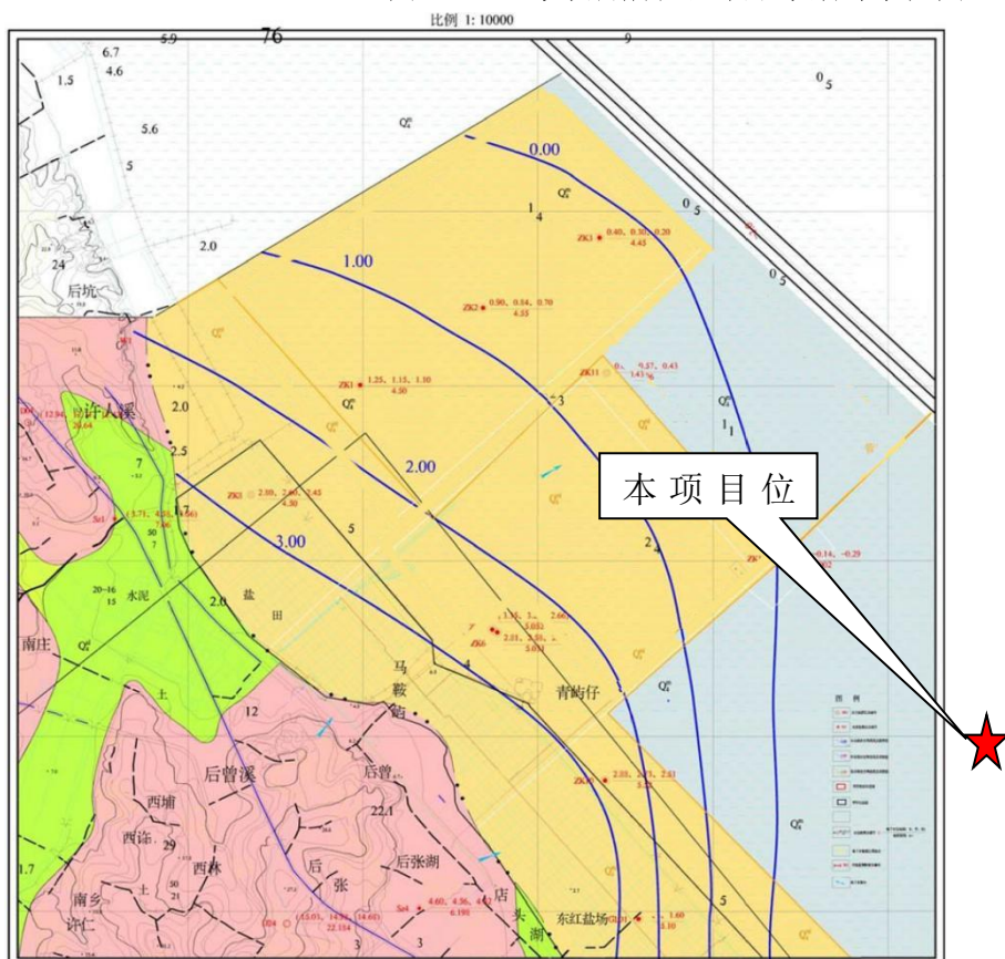
图 6.3-5 本项目所在区域平水期等水位图
