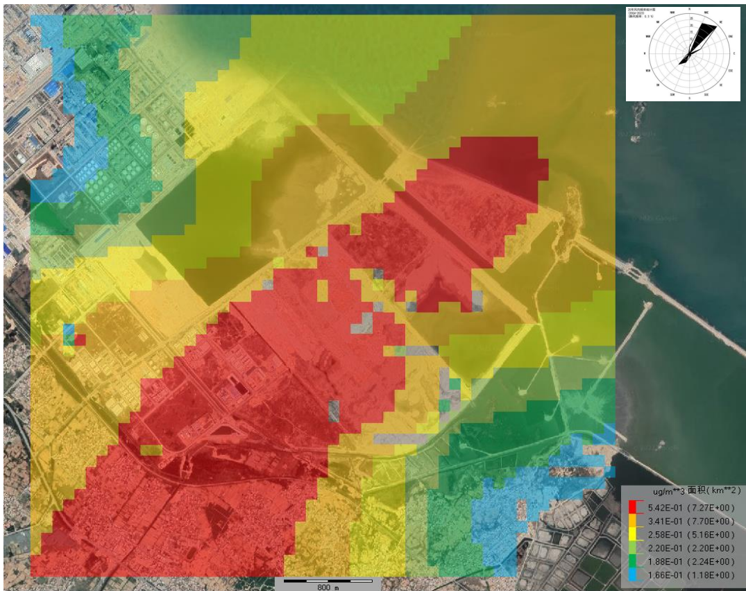
图 6.2-10 NO 2 年均浓度网格分布图
