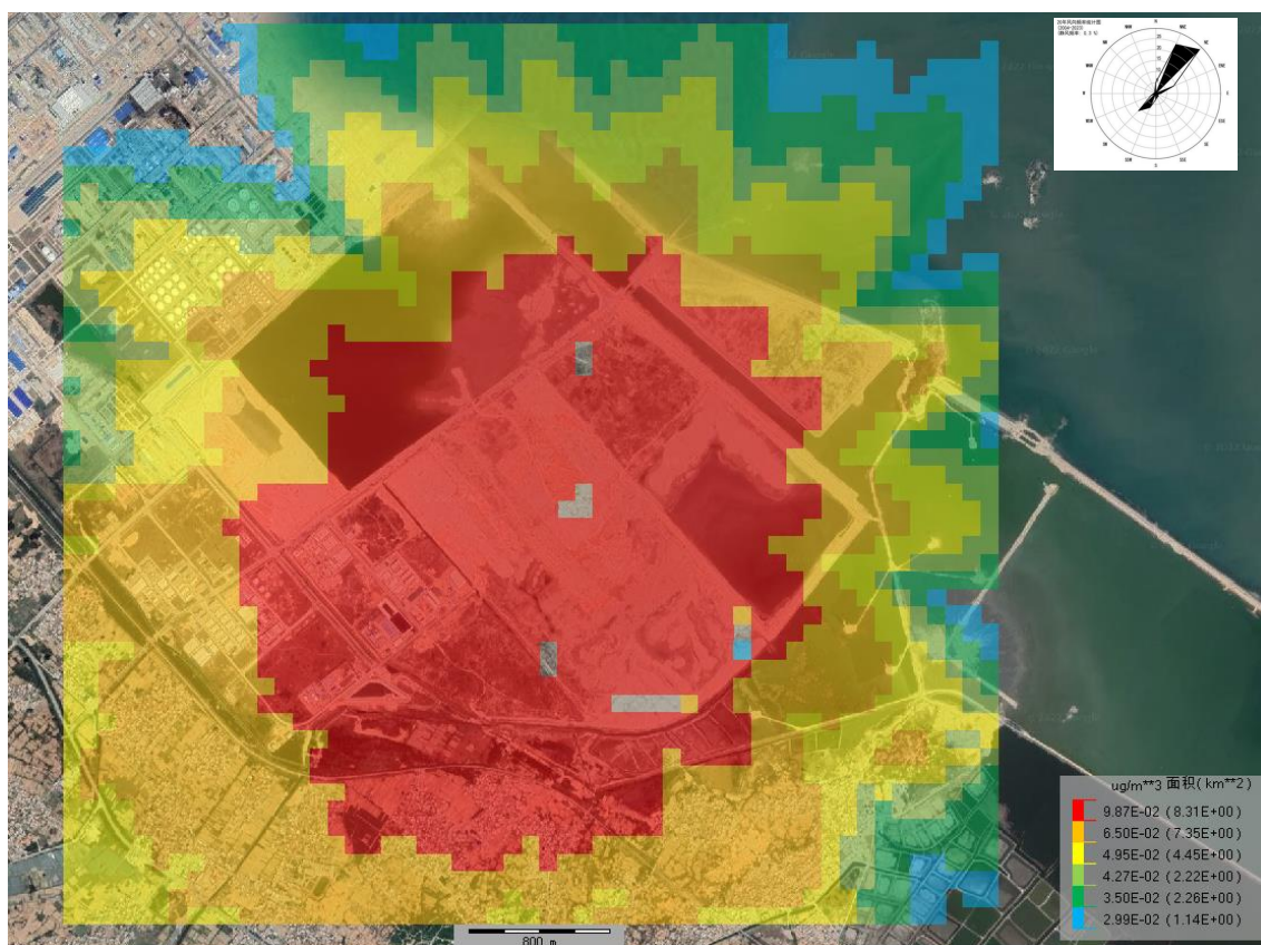
图 6.2-12 硫化氢最大小时平均浓度网格分布图
