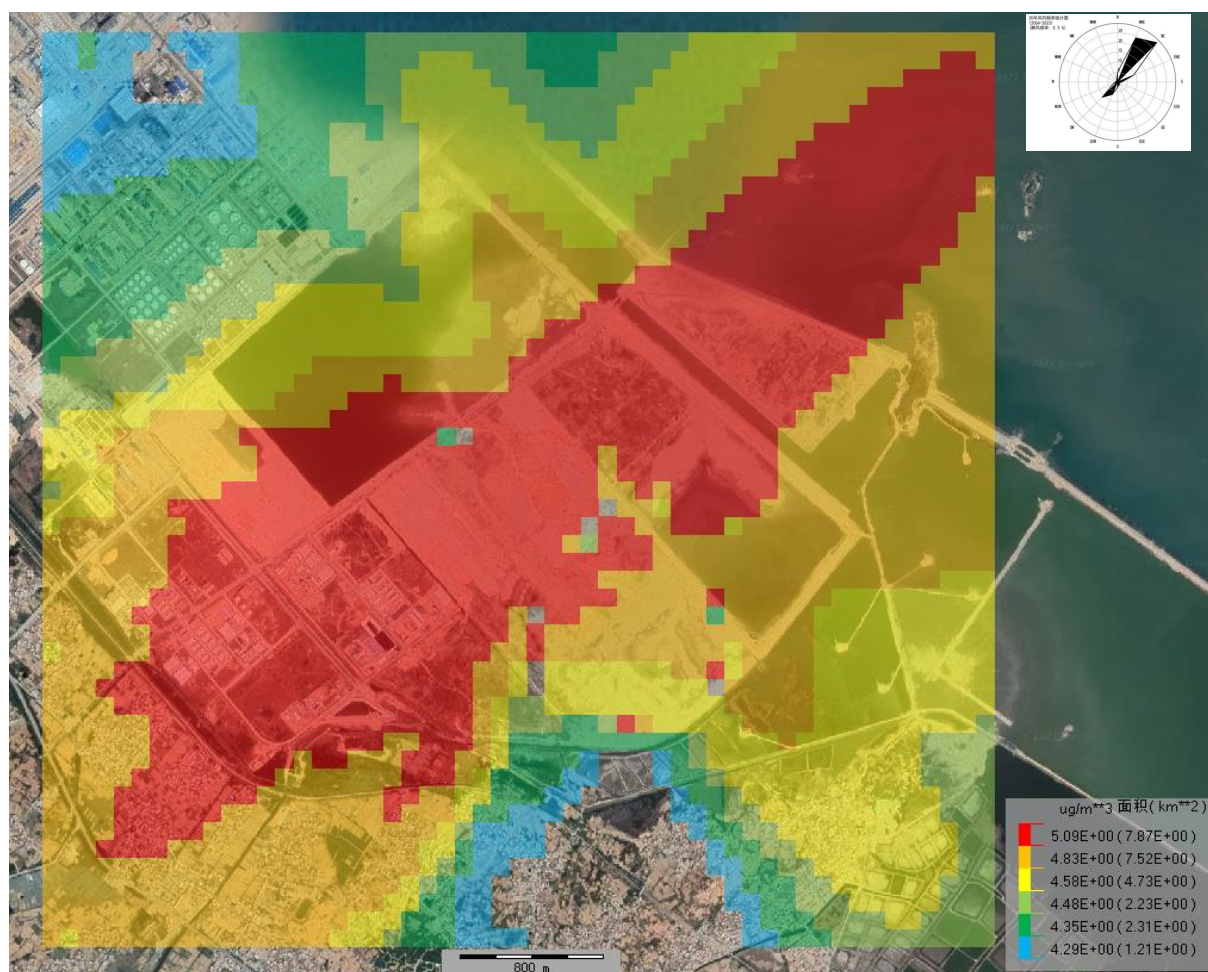
图 6.2-15 SO 2 叠加在建拟建和现状背景保证率下日平均浓度网格分布图
