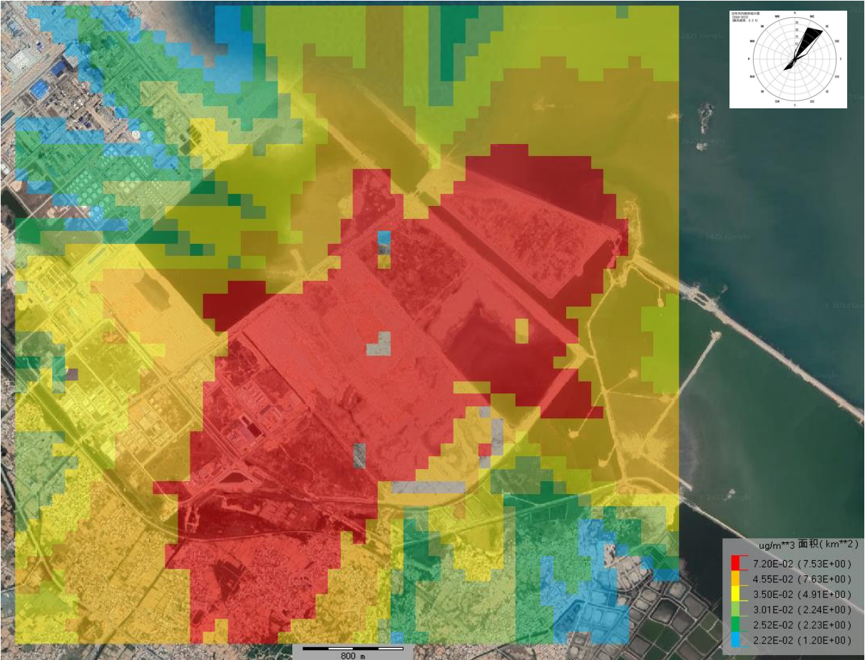
图 6.2-14 硫酸日平均浓度网格分布图
