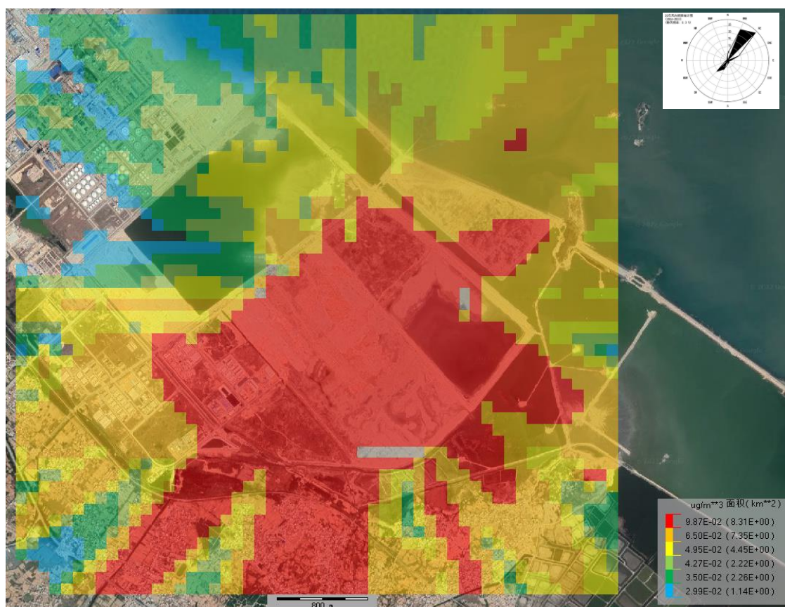
图 6.2-13 硫酸最大小时平均浓度网格分布图
