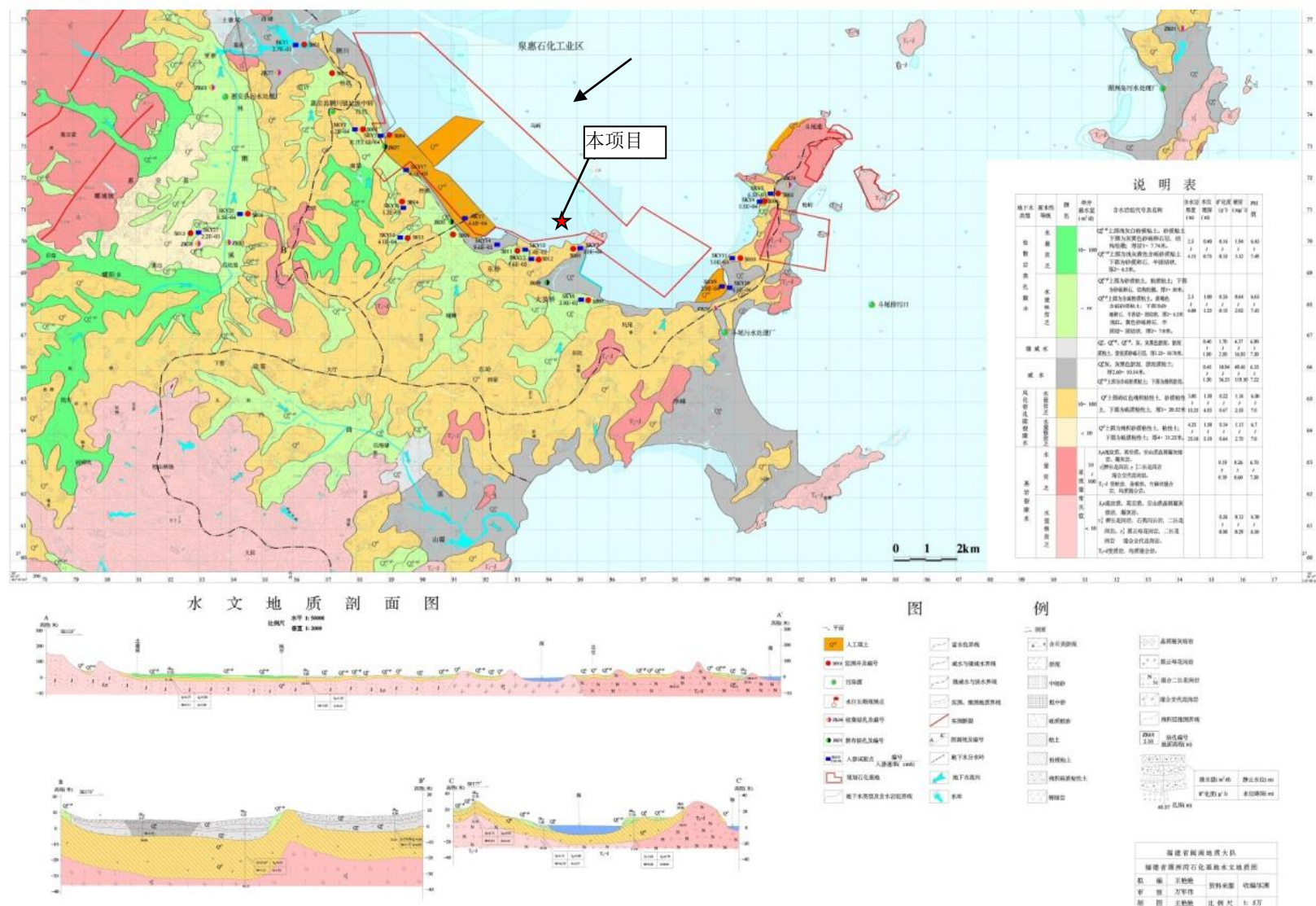
图 6.3-1 评价区域地质地貌图
