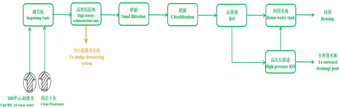
图 8.2-3 清净废水处理系统工艺流程图
