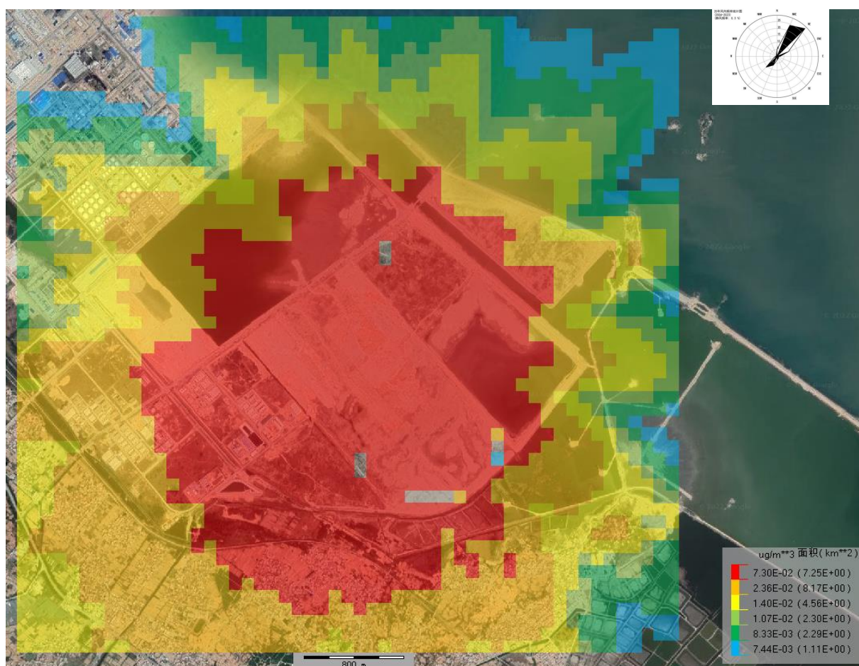
图 6.2-11 NMHC 最大小时平均浓度网格分布图
