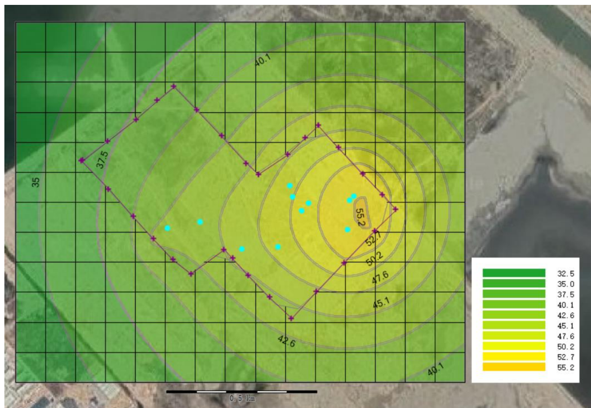
图 6.4-2 本项目叠加厂内拟建在建噪声污染源运营期噪声值预测图
