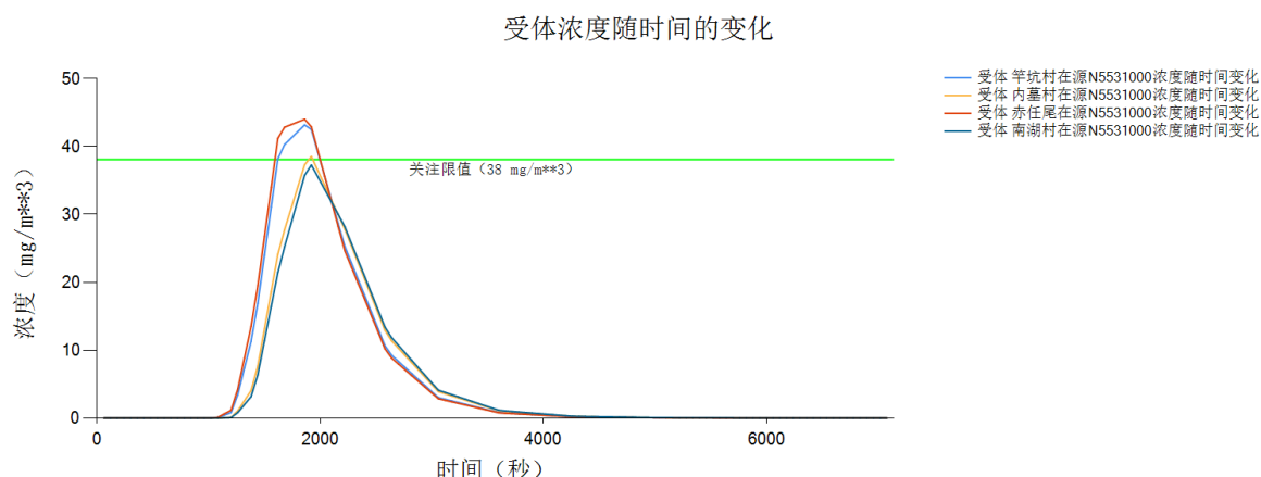
图 7.5-2 硫化氢泄漏事故关心点浓度随时间的变化曲线（最不利气象条件）
