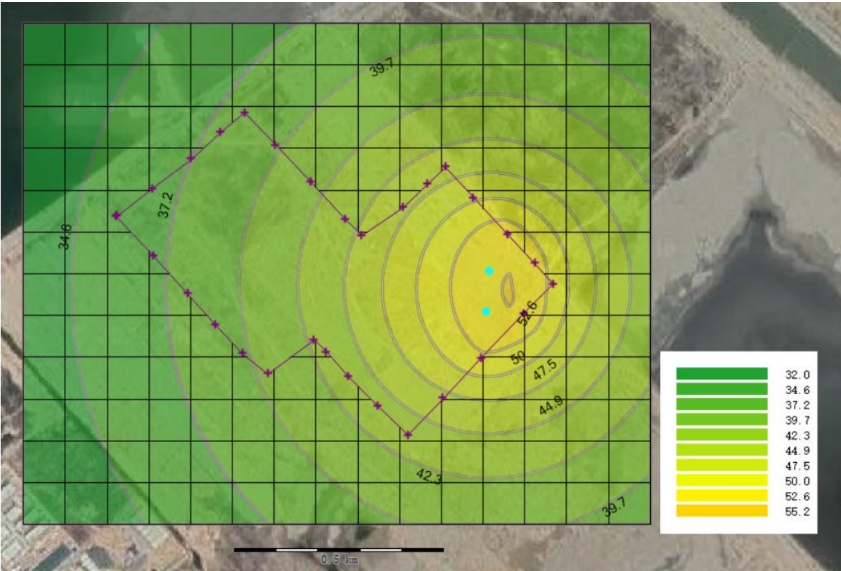
图 6.4-1 本项目新增噪声污染源运营期噪声贡献值预测图
