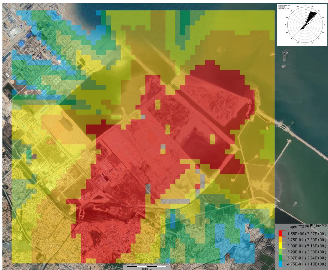
图 6.2-7 SO 2 最大日平均浓度网格分布图
