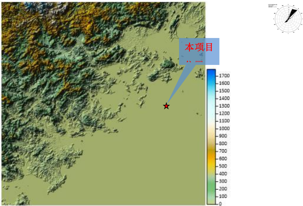
图 6.2-3 预测范围内地形高程等值线图
