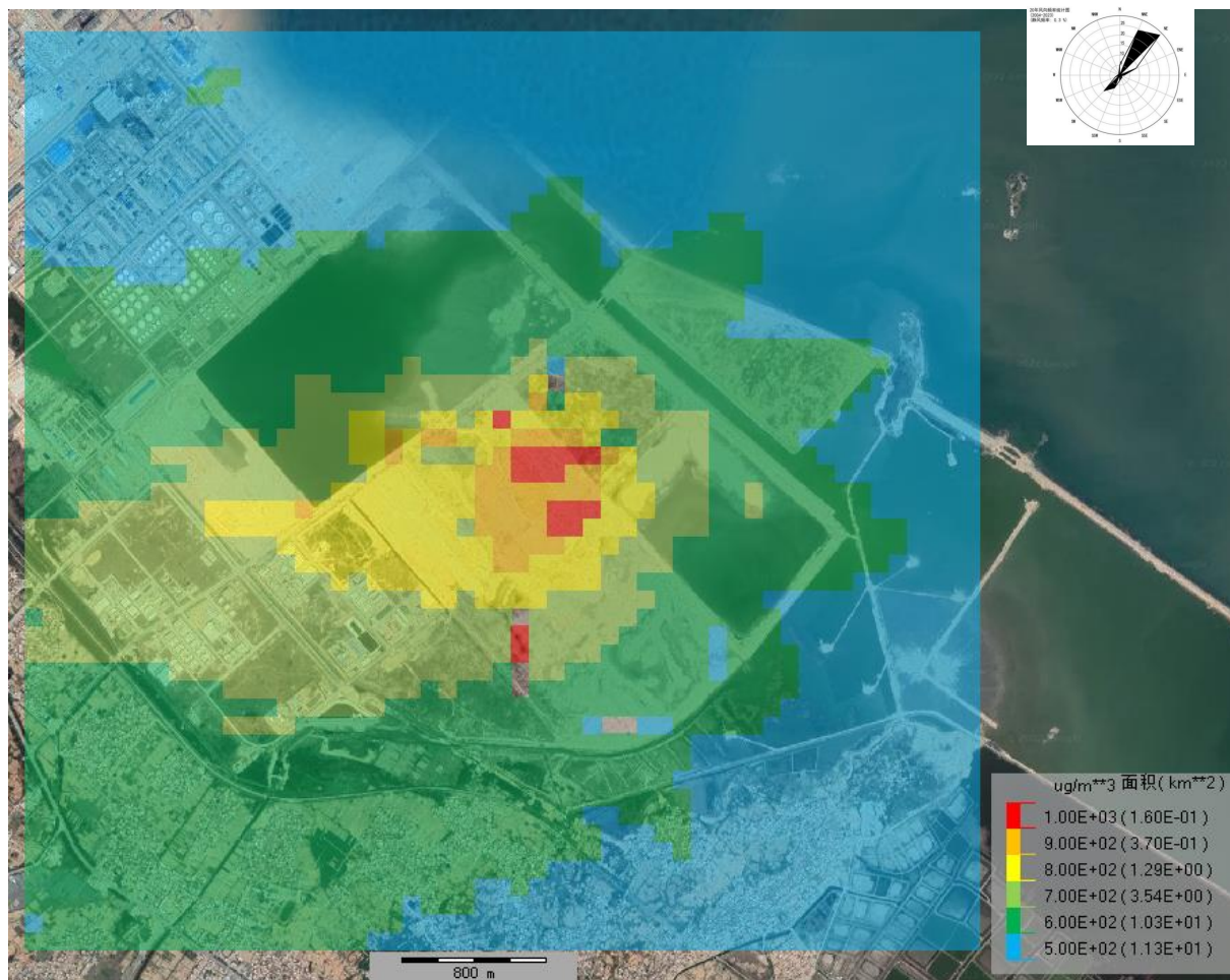
图 6.2-19 NMHC 叠加在建拟建和现状背景值后小时平均浓度网格分布图
