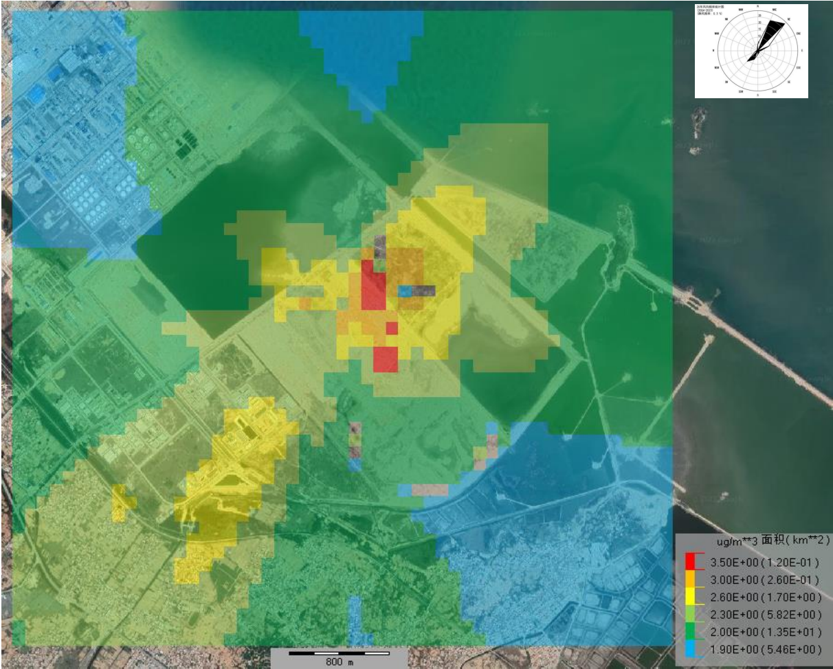
图 6.2-22 硫酸叠加在建拟建和现状背景值后日平均浓度网格分布图
