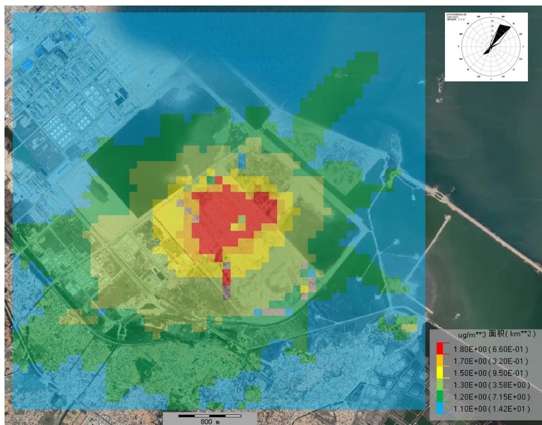
图 6.2-20 硫化氢叠加在建拟建和现状背景值后小时平均浓度网格分布图
