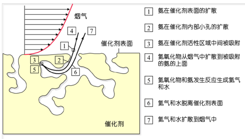
图 8.2-1 SCR 脱硝原理示意图
