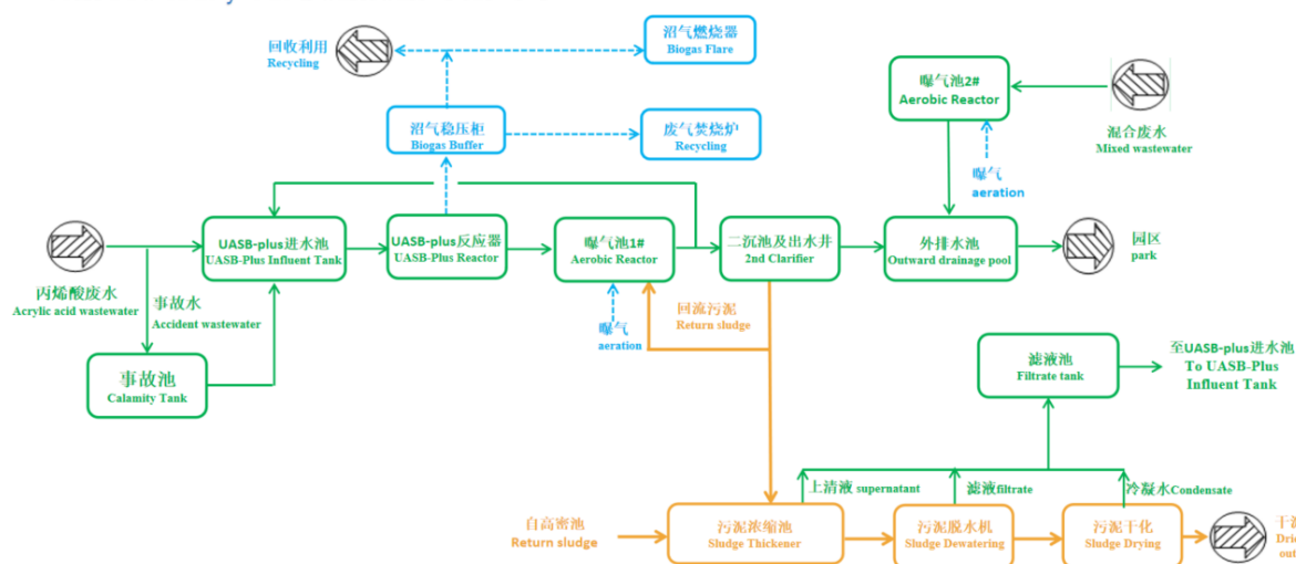
图 8.2-2 混合废水处理系统工艺流程图
