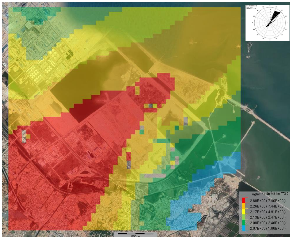
图 6.2-16 \text{SO}_2 叠加在建拟建和现状背景后年均浓度网格分布图
