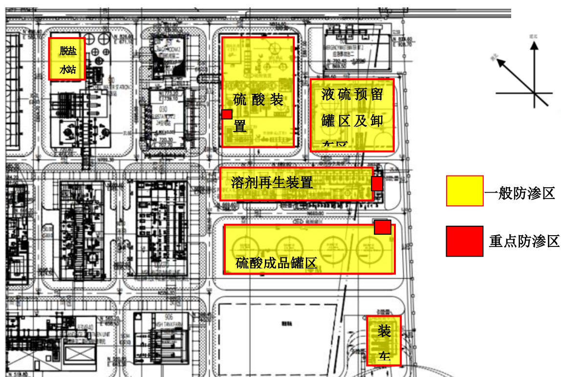
图 8.2-4 地下水分区防渗示意图
