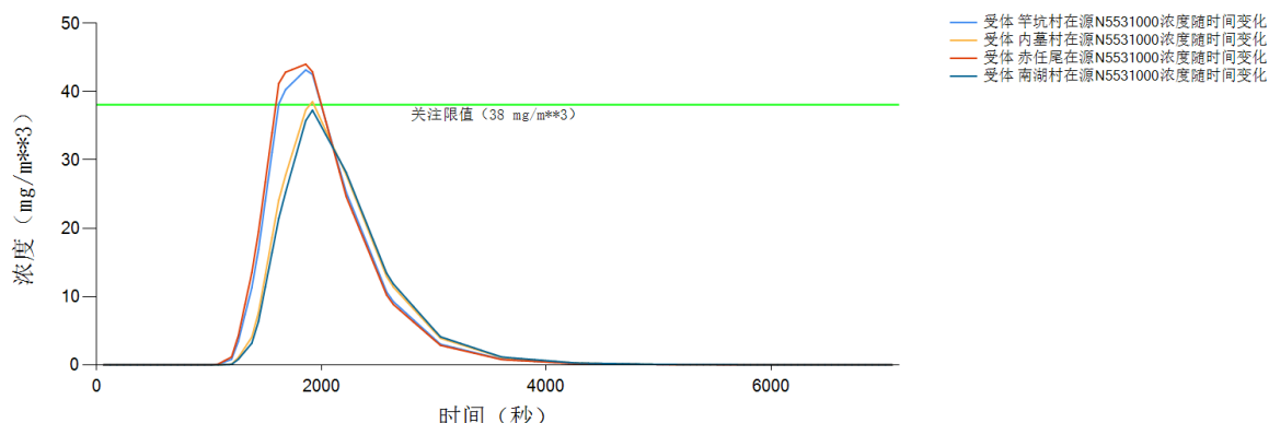
图 7.5-2 硫化氢泄漏事故关心点浓度随时间的变化曲线(最不利气象条件)
