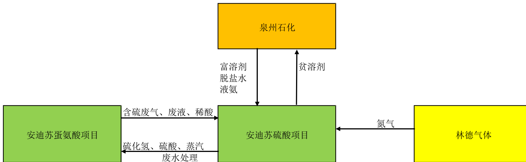
图 4.1-1 本项目与园区周边企业/项目原辅材料联系示意图
