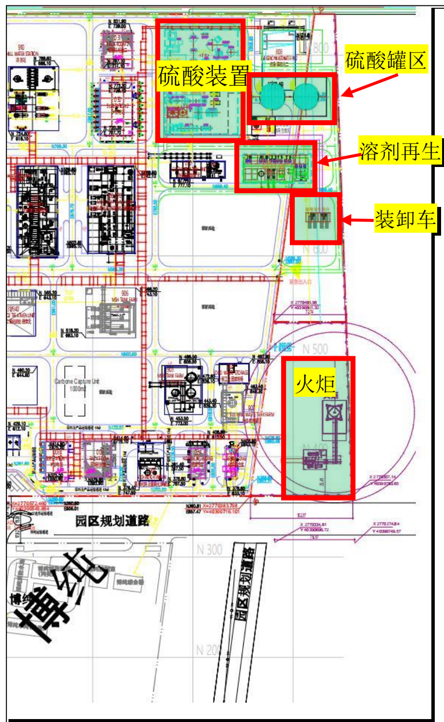
图 4.1-2 总平面布置图
