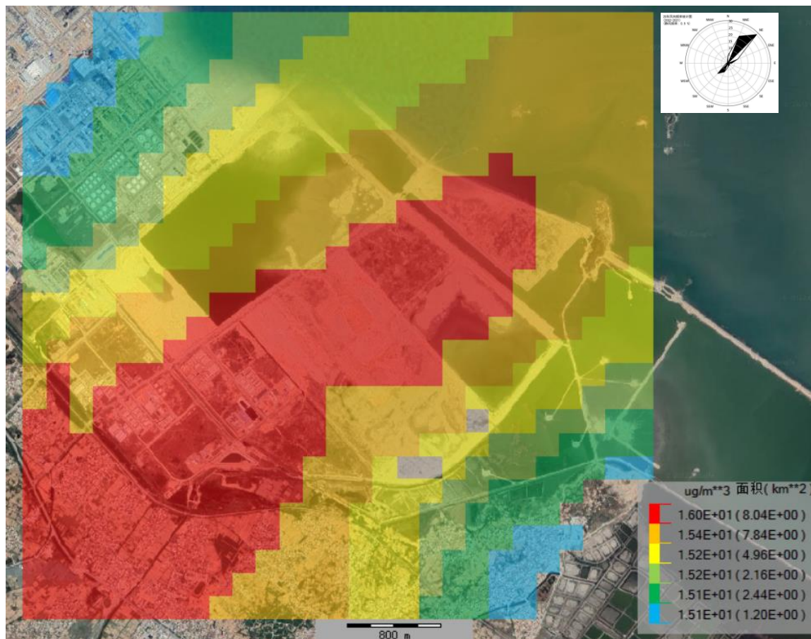
图 6.2-28 NO 2 叠加在建拟建和现状背景后年均浓度网格分布图
