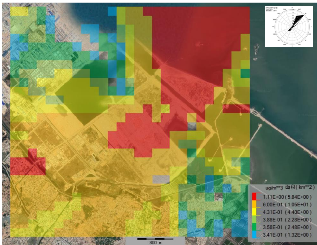
图 6.2-37 硫化氢叠加在建拟建和现状背景值后小时平均浓度网格分布图
