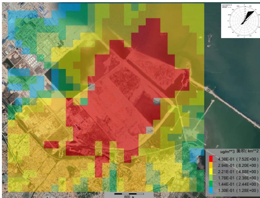
图 6.2-16 CO 最大日均浓度网格分布图
