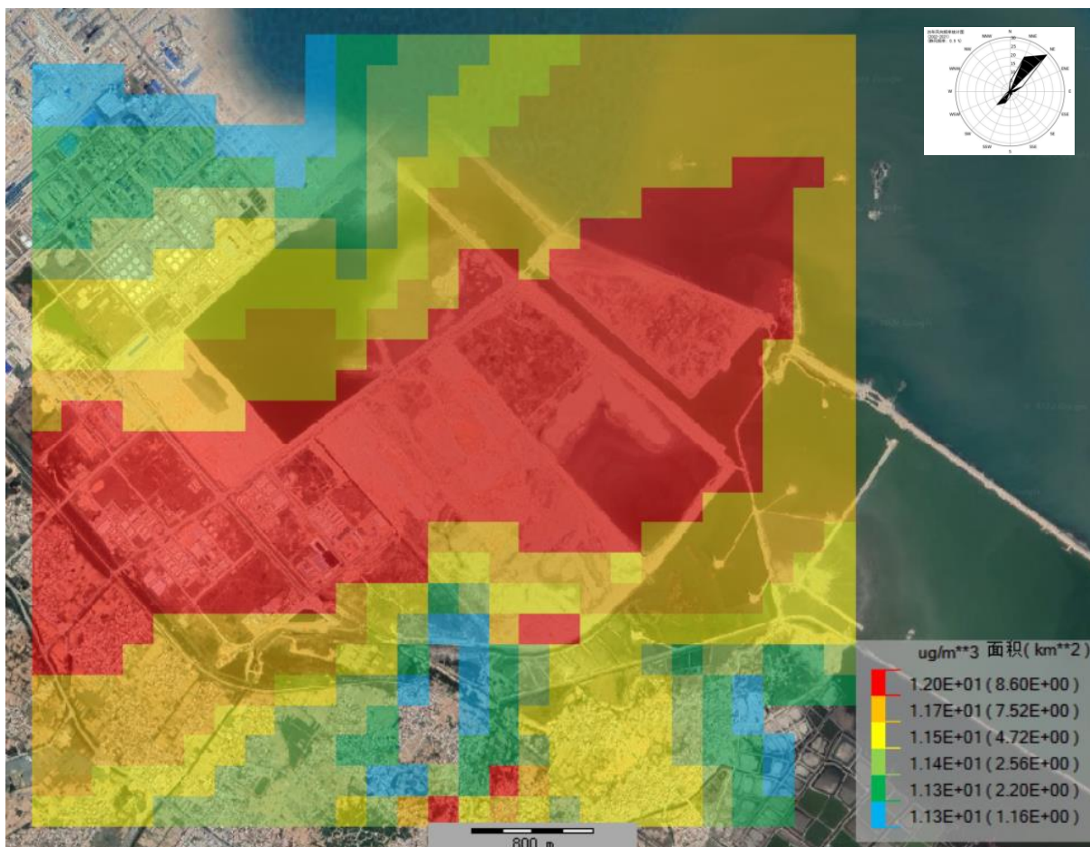
图 6.2-25 SO 2 叠加在建拟建和现状背景保证率下日平均浓度网格分布图
