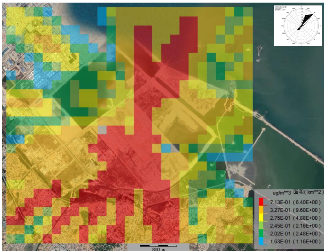
图 6.2-18 丙烯醛最大小时平均浓度网格分布图
