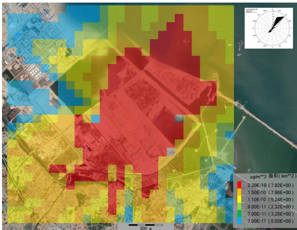
图 6.2-41 二噁英叠加在建拟建和现状背景值后日平均浓度网格分布图
