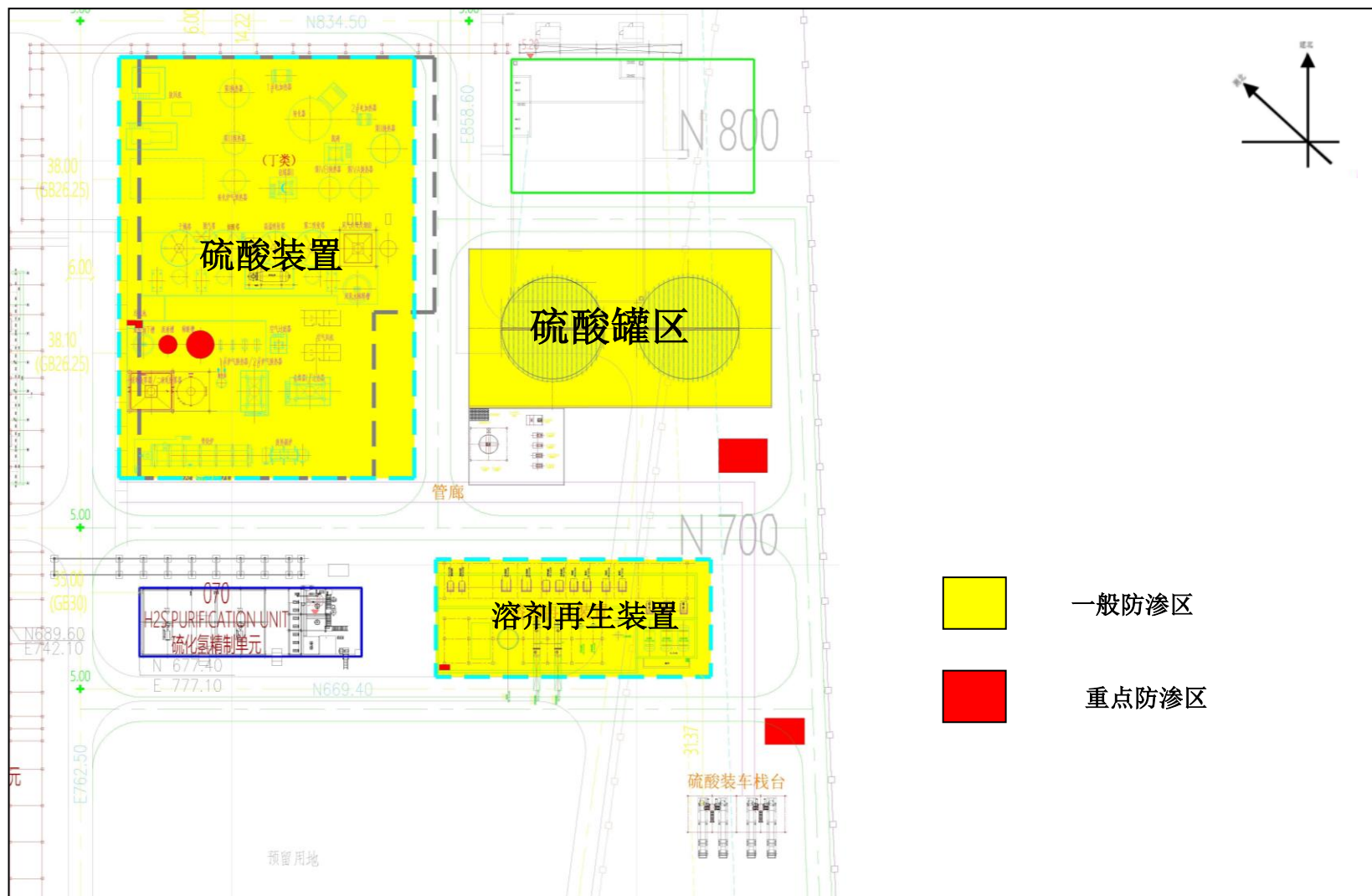
图 8.2-3 地下水分区防渗示意图
