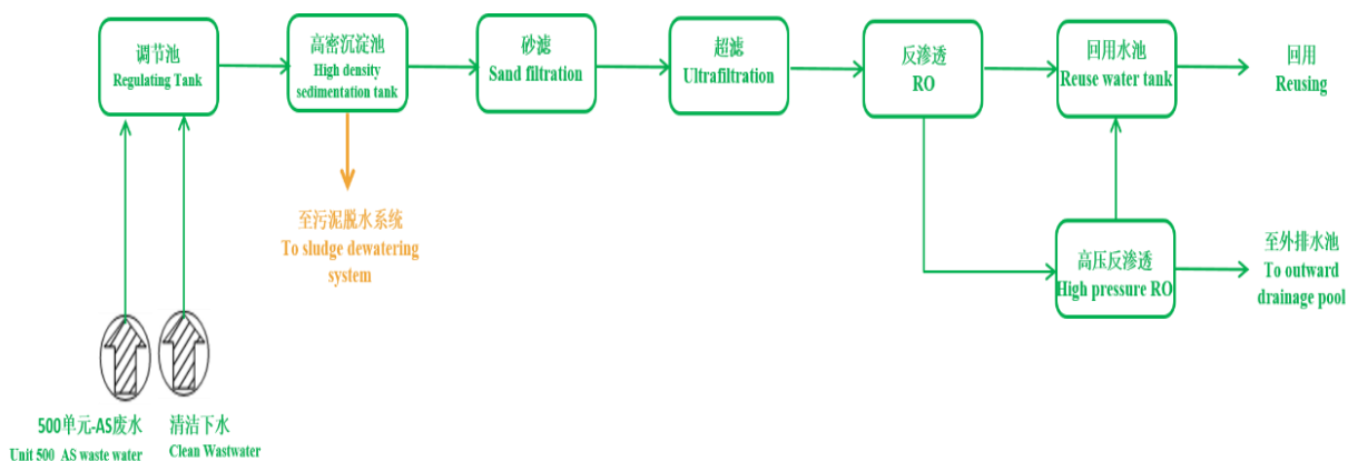
图 8.2-2 清净废水处理系统工艺流程图
