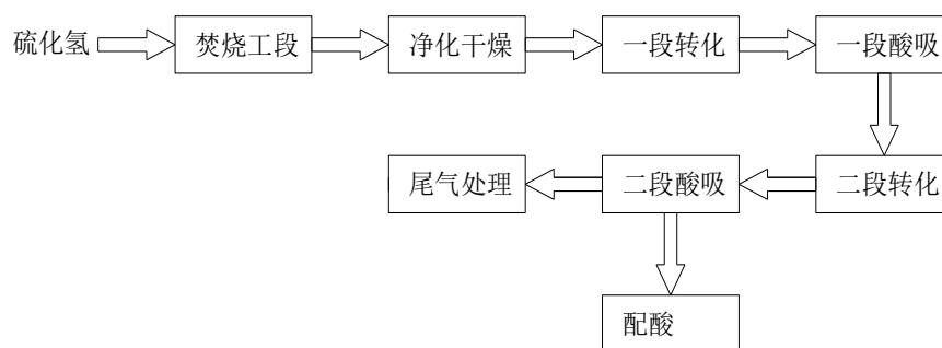
图 4.3-3 干法制硫酸生产工艺路线图
