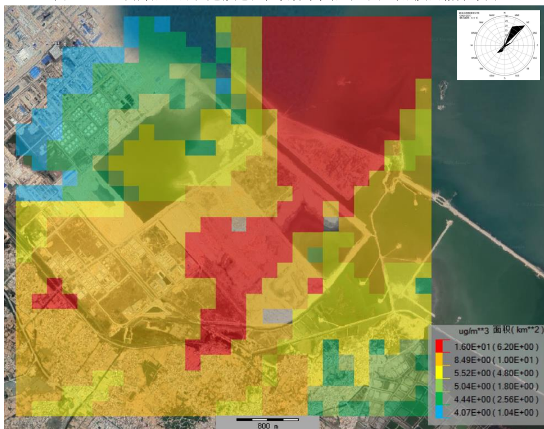
图 6.2-36 甲醇叠加在建拟建和现状背景值后小时平均浓度网格分布图
