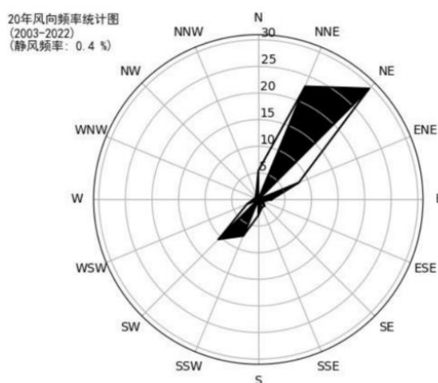
图 6.2-2 崇武风向玫瑰图 (静风频率 0.4%)
