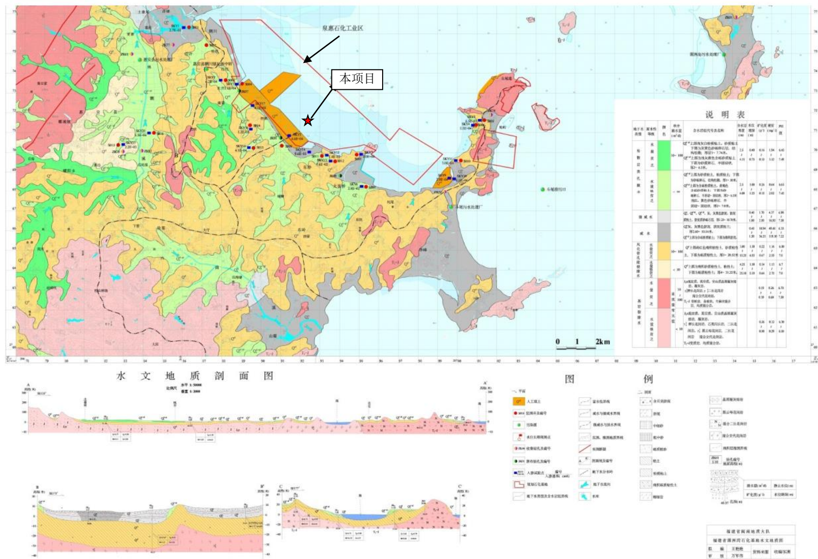
图 6.3-1 评价区域地质地貌图
