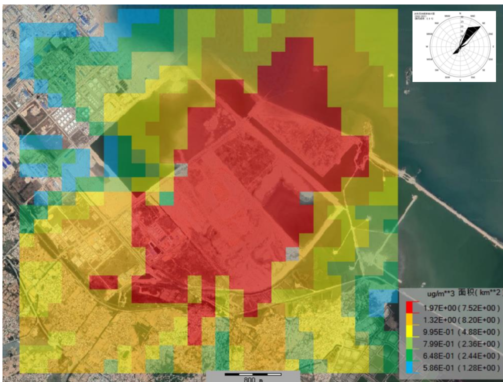
图 6.2-9 NO 2 最大日平均浓度网格分布图
