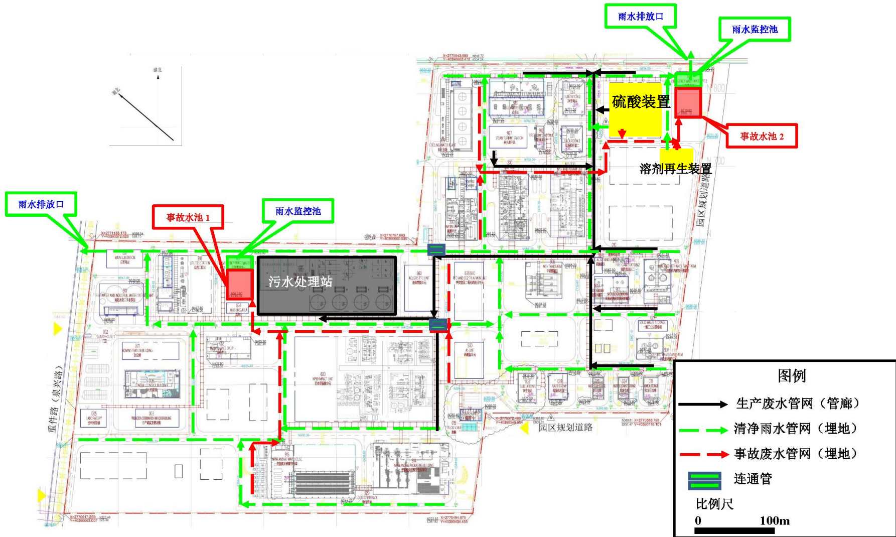
图 4.4-1 排水系统管网示意图
